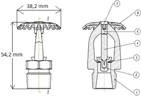
Upright
